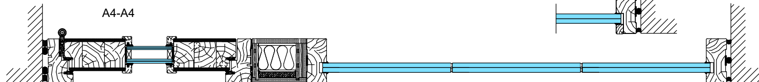
Lasiaukollinen ovi sisäänaukeava, sähköpieli
