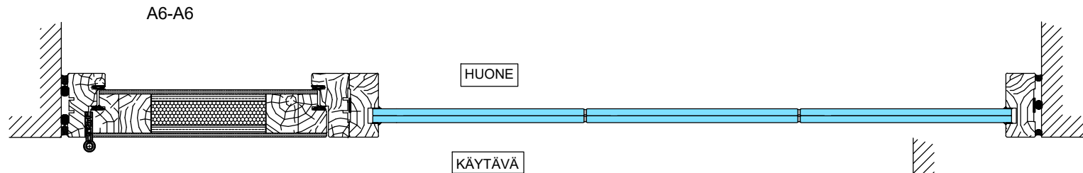
Umpiovi ulosaukeava, apukarmi
