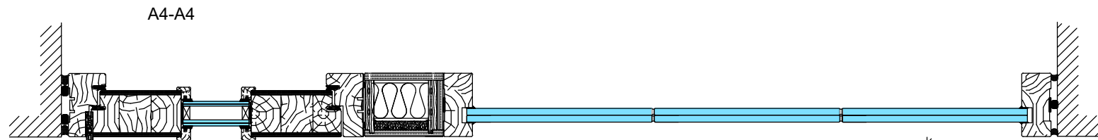
Lasiaukollinen ovi ulosaukeava, sähköpieli
