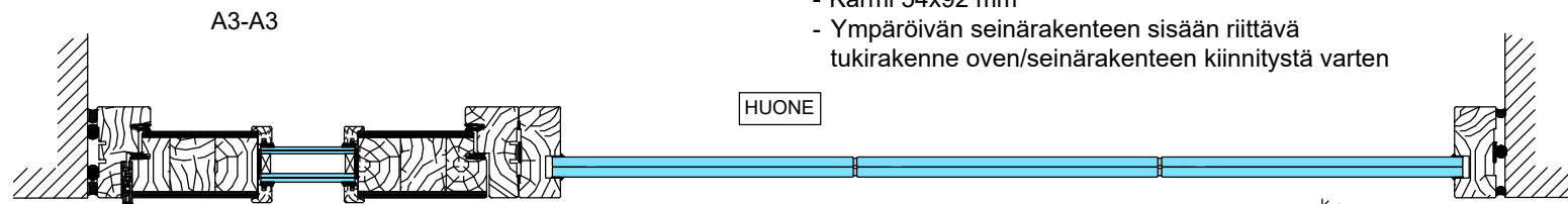
Lasiaukollinen ovi ulosaukeava, apukarmi
