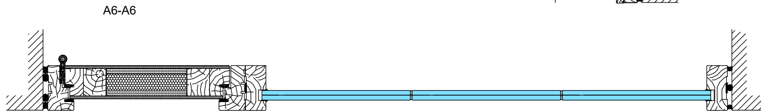
Umpiovi sisäänaukeava, apukarmi
