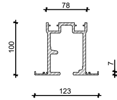
Yläpalkki
