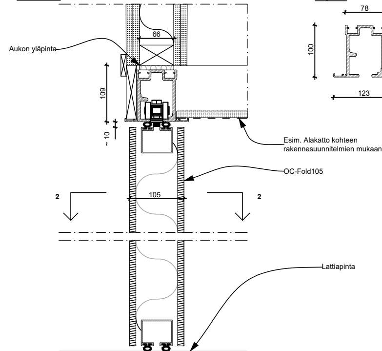
Leikkaus 1-1
